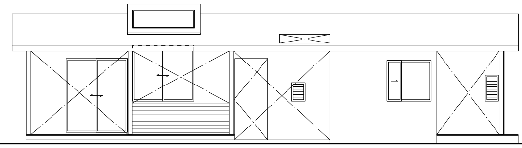
南立図
