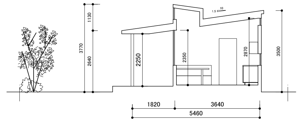
断面図
