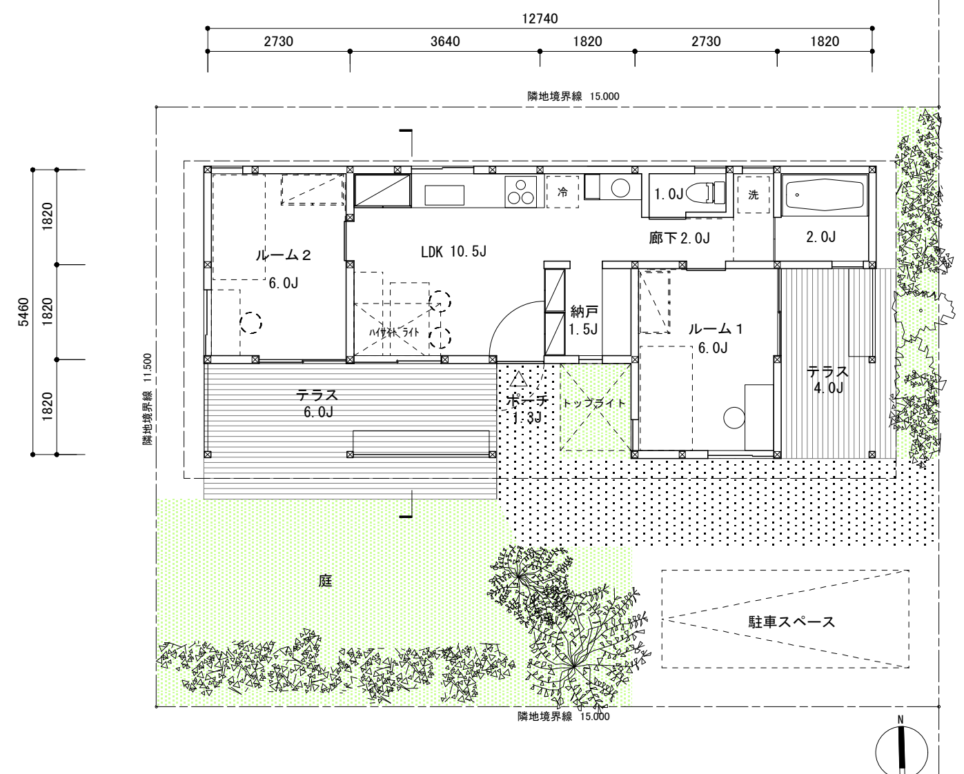
配置図兼平面図 S=1:100
