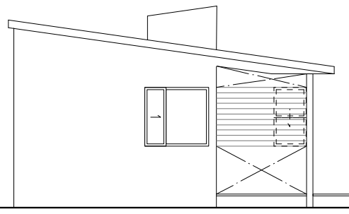
西立図
